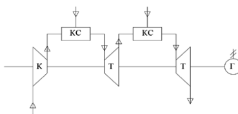
Рис. 2. Часть схемы СО2-цикла с одноступенчатым перегревом рабочего тела. Обозначения: КС – камера сгорания, К – компрессор, Т – турбина, Г – генератор.
