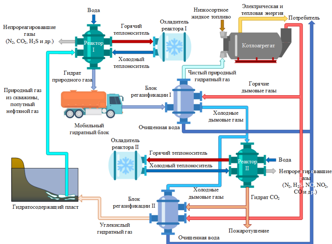
Рис. 1. Концептуальная схема применения газогидратных технических решений в энергетических приложениях на основе анализа результатов исследований [1-3].
