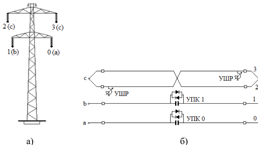
Рис. Промежуточная опора и схема ЧТЛ: а - промежуточная опора; б - схема ЧТЛ
