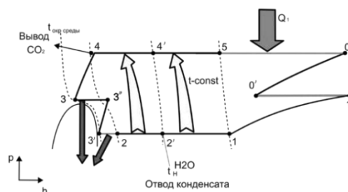
Рис. 1. Термодинамический CO 2 -цикл с одноступенчатым перегревом рабочего тела
