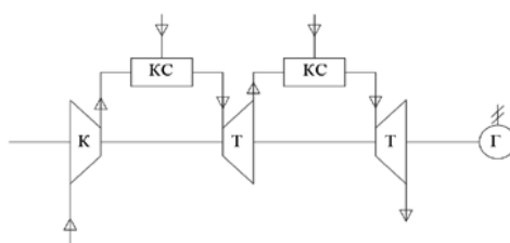
Рис. 2. Часть схемы CO 2 -цикла с одноступенчатым перегревом рабочего тела. Обозначения: КС – камера сгорания, К – компрессор, Т – турбина, Г – генератор.
