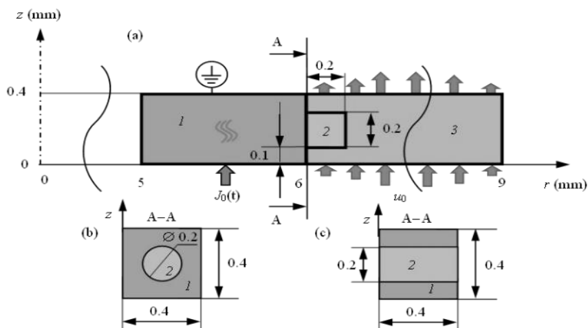
Рисунок 2. Область расчета. 1 – нагреватель, 2 – выступ на поверхности нагревателя, 3 – поток воды. (a) – осесимметричная расчетная модель; (b) – поверхность нагревателя в физическом эксперименте; (c) – поверхность нагревателя в осесимметричной модели.
