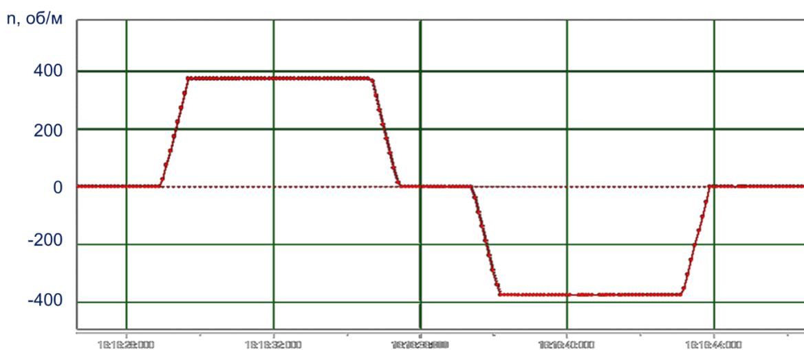
Рис. 2. Экспериментальная циклограмма работы механизма Е перемещения крана
